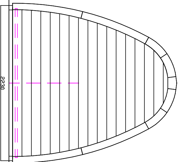
Rückansicht
