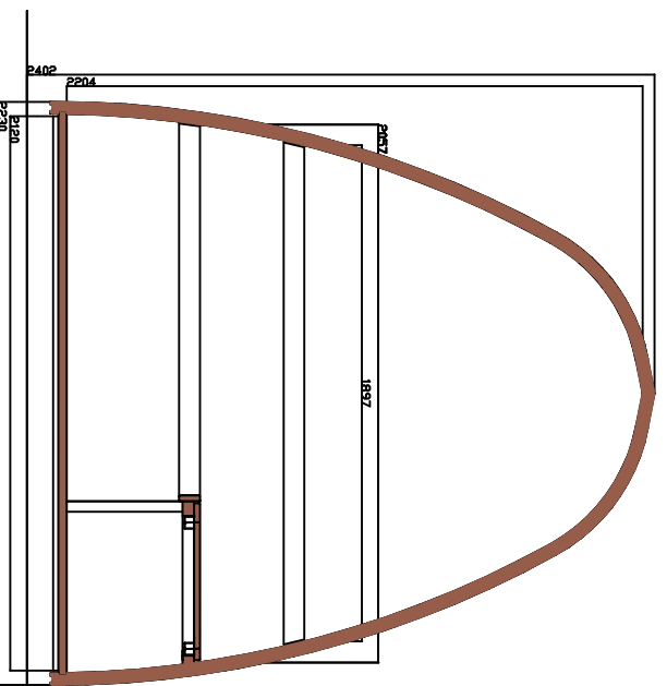
Schnitt
